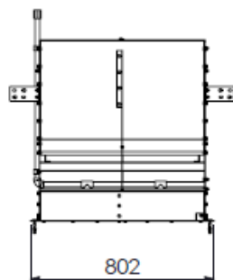
COMED. SUINO TERMINAÇÃO INOX 2 BOCAS DUPLO
