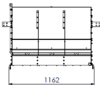
COMED. SUINO TERMINAÇÃO INOX 3 BOCAS DUPLO
