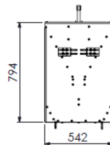
COMED. SUINO TERMINAÇÃO INOX 2 BOCAS DUPLO
